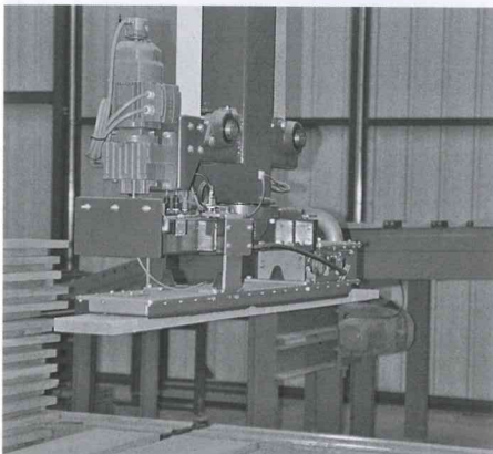
Exakte Positionierung: Der Greifer kann mehrere Ablagepositionen einspeichern
